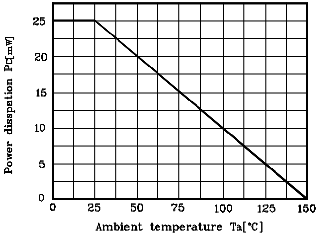
Fig. 1 P_C - T_a
