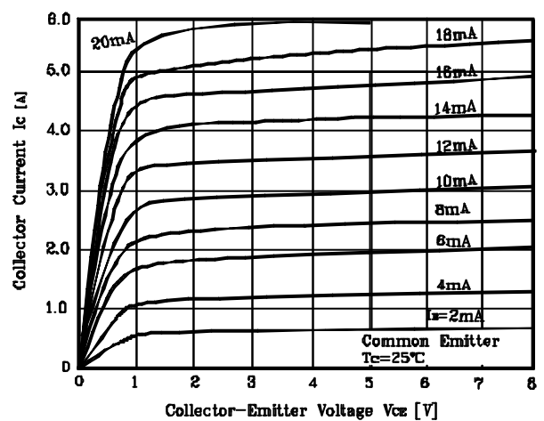
Fig. 4 I_C - V_{CE}
