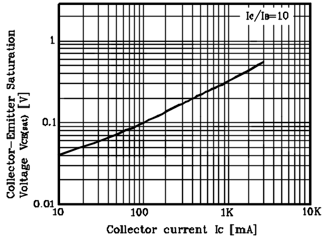
Fig. 2 V_{CE(sat)} - I_C
