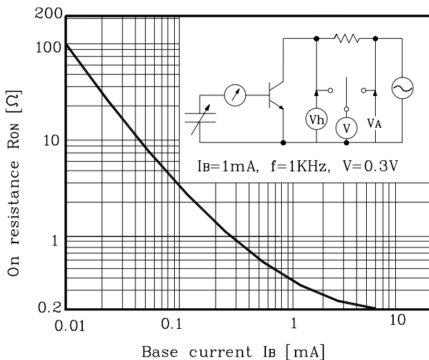
Fig. 5 R_{ON} - I_B
