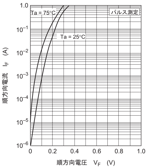
図1. 順方向特性
