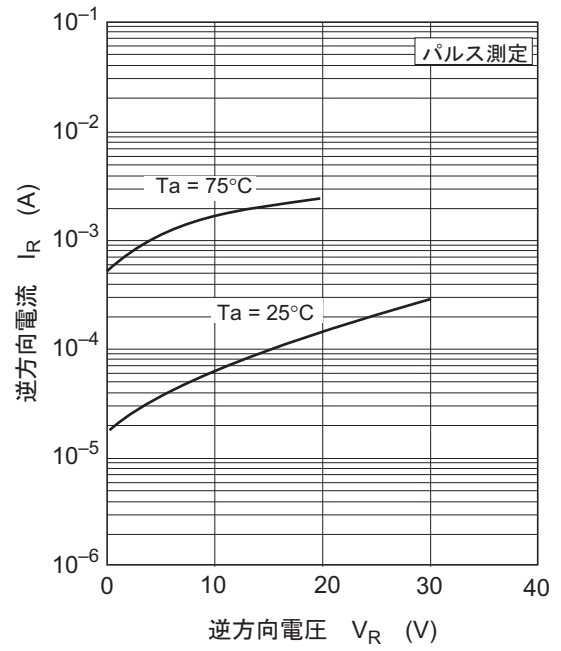
図2. 逆方向特性
