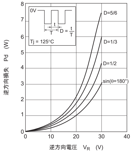
图5. 逆方向損失 对 逆電圧特性
