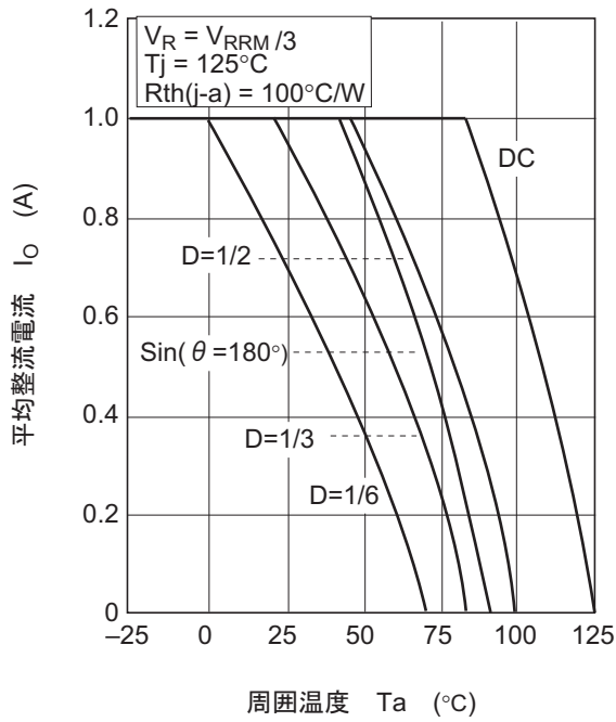
图6. 平均整流電流 对 周圍温度特性
