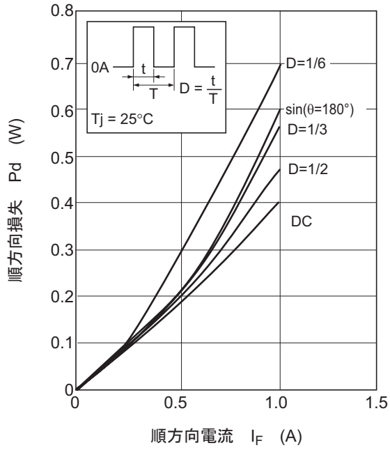
图4. 順方向損失 对 順電流特性
