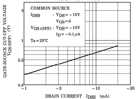
VGS(OFF) - IDSS
